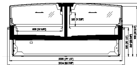
M. 1875 | 2500 | 3125 | 3750 mm
